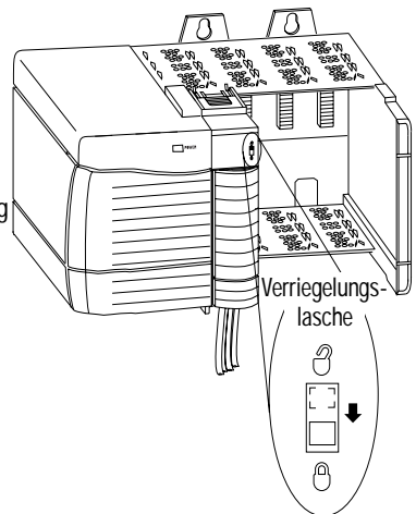
Die RTB schnell und gleichmäßig gegen das Modul drücken, bis die Laschen einrasten.
