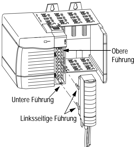
Die obere, untere und linke Seitenführung der RTB mit den Führungen auf dem Modul ausrichten.
