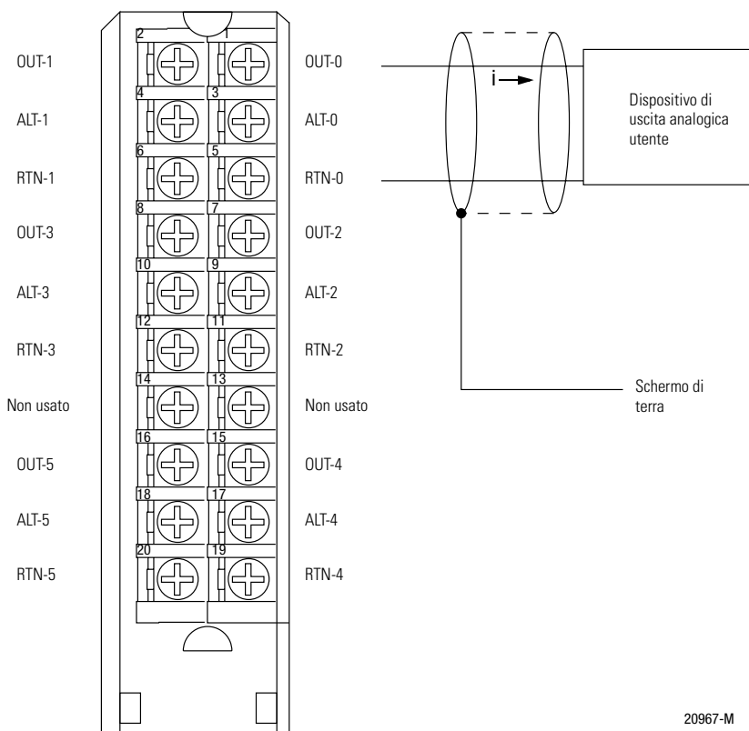
Esempio di cablaggio del 1756-OF6CI per carichi di 0-550Ω
