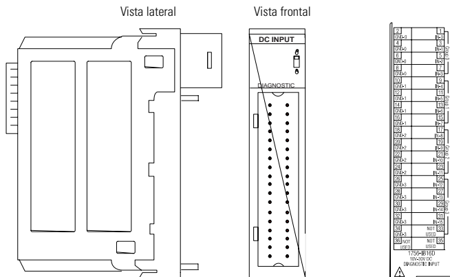
Módulo 1756-0B16D
