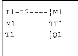
Diagrama de circuito Pico
