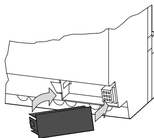
1760-MM1 para todos los controladores 1760-L12xxx
