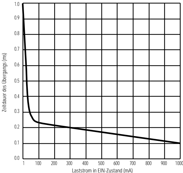
Dauer des Übergangsimpulses als Funktion des Laststroms
