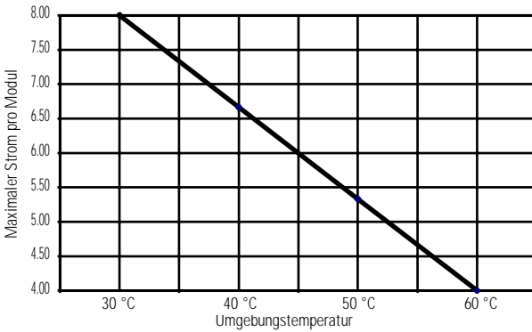
1769-OV16 Maximaler Strom pro Modul vs. Temperatur
