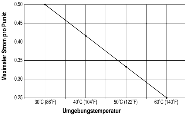
1769-OA8 Maximaler Strom pro Punkt in Abhängigkeit von der Temperatur
