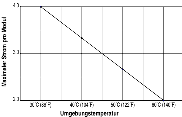
1769-OA8 Maximaler Strom pro Modul in Abhängigkeit von der Temperatur
