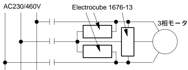
図11 標準的なサージ抑制アプリケーション
