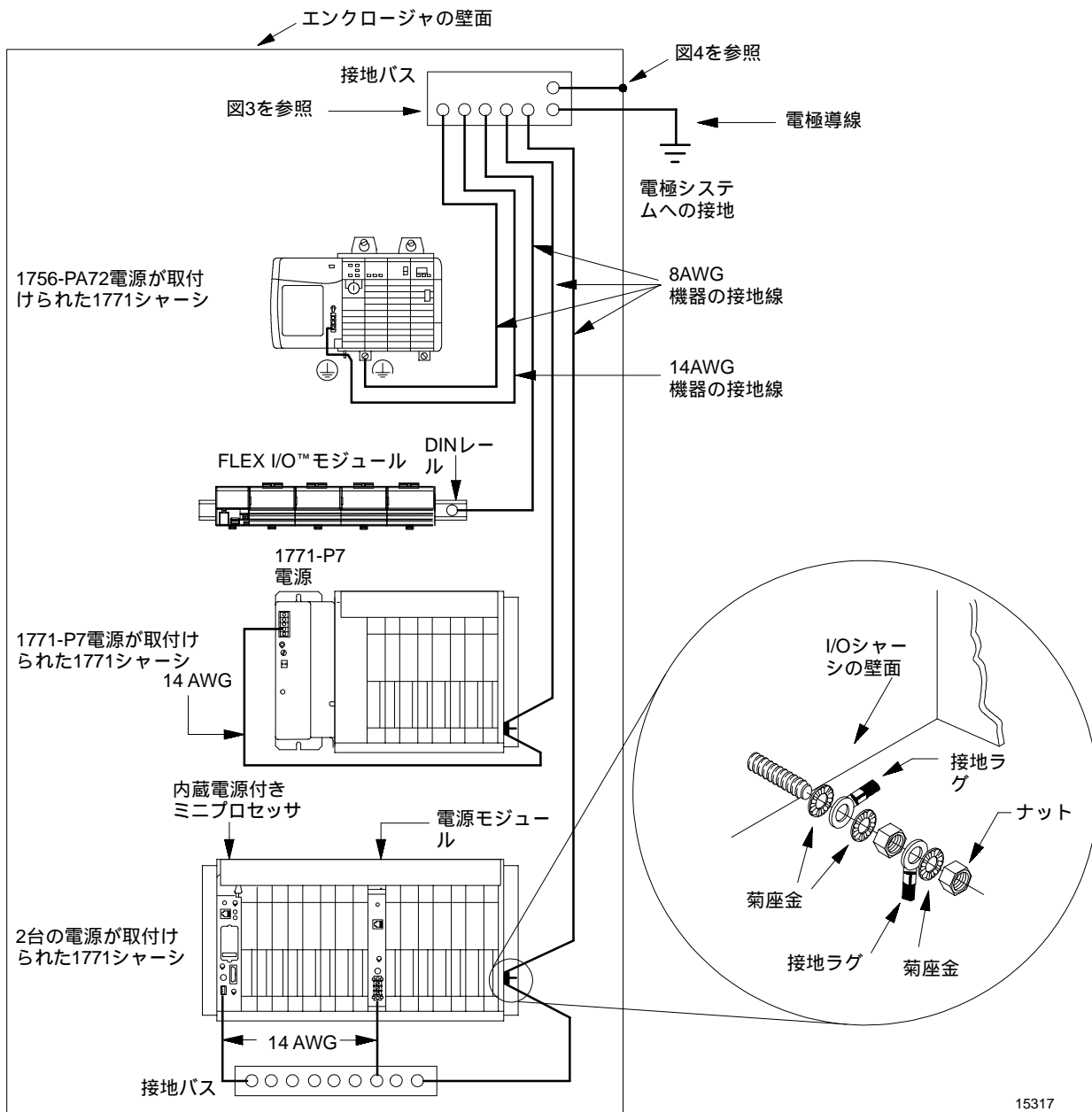
図6 標準的な接地構成
