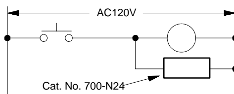
図11 標準的なサージ抑制アプリケーション
