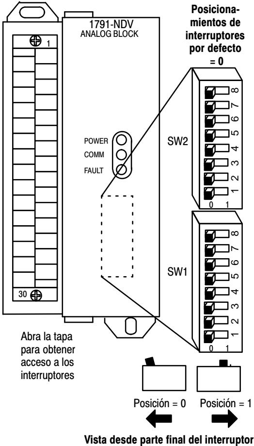
Figura 7 Posicionamiento de los interruptores
