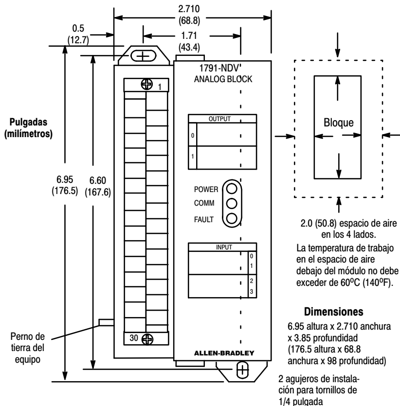
Figura 1 Dimensiones de montaje para el módulo de bloque de E/S analógica Cat. No. 1791-NDV
