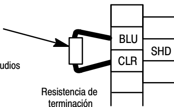
Figura 8 Instalación de la resistencia de terminación
