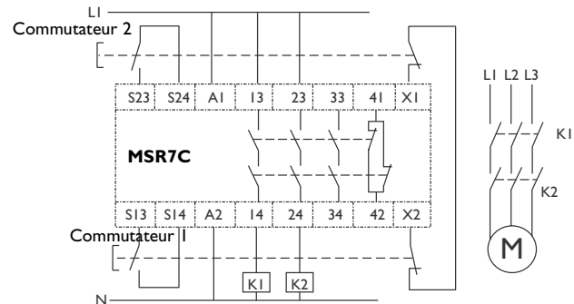
Commande bimanuelle deux voies, réarmement automatique, sortie deux voies, sortie non surveillée
